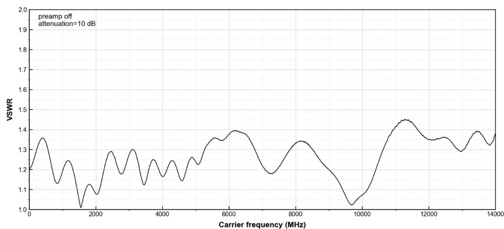
VSWR
