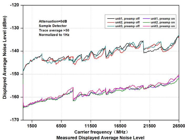
DANL
