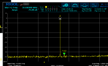
-70 dBc SFDR
